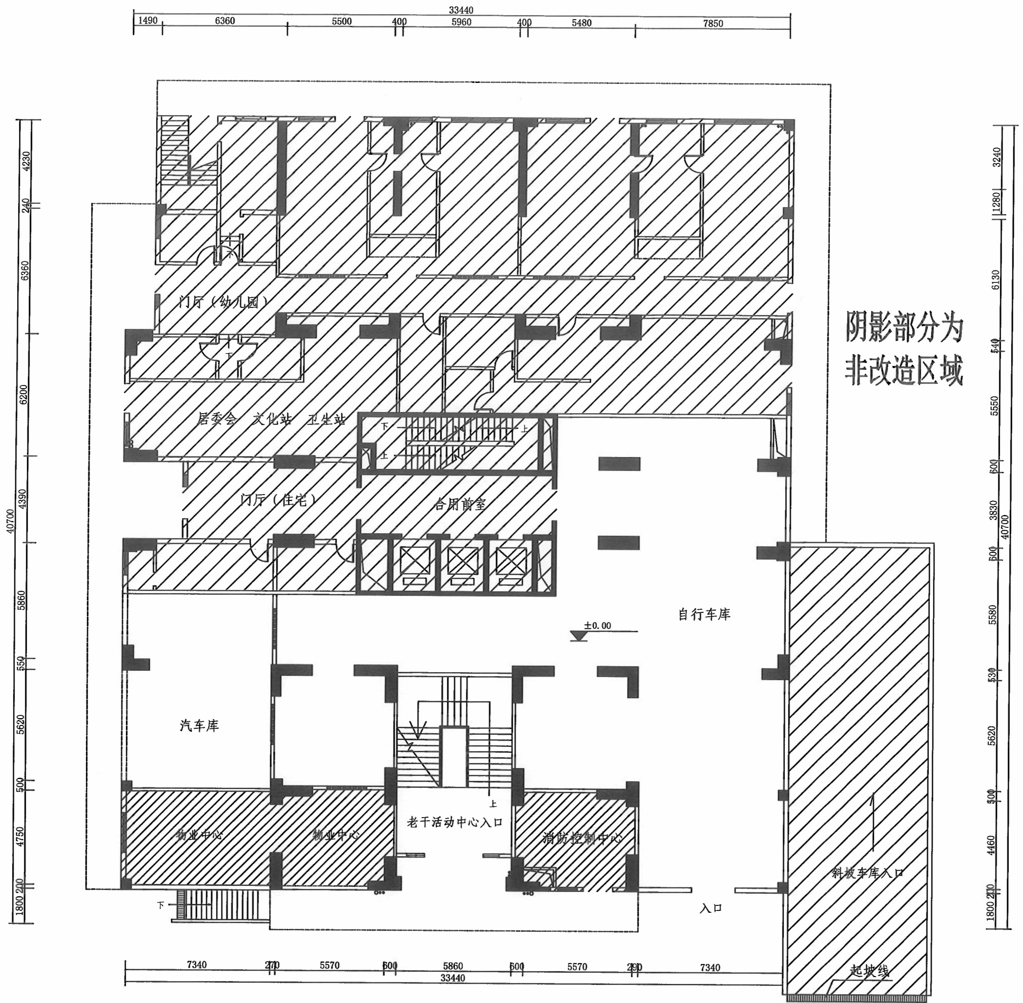
云鹤轩1F原始结构图
